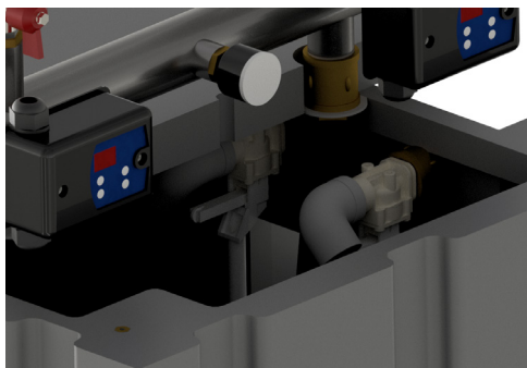
Detail: Ansicht Zulauf Break 7 Typ AB
