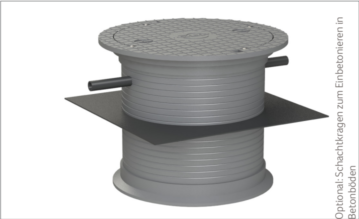
Optional: Einkürzbares Verlängerungselement
