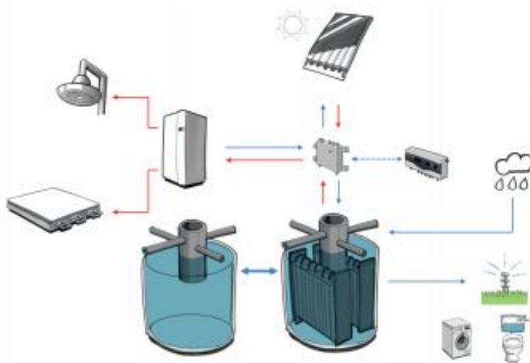
Funktionsschema der thermodynamischen Regenwassernutzung
