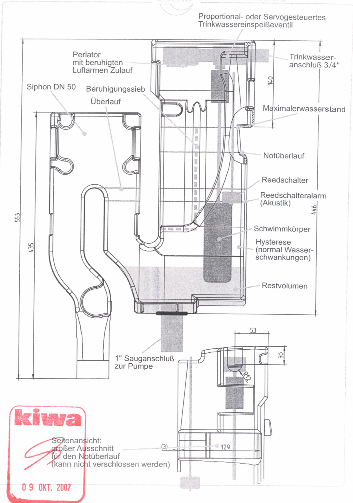
Figuur: detail van binnenwerk GEP Rainmanager, beveiliging familie A, type B
