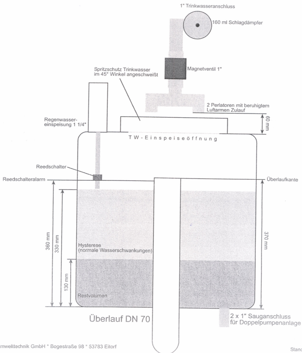
Figuur: detail van binnenwerk GEP C-Class, beveiliging familie A, type A
